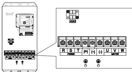
Рис.4-13 37~55кВт клеммы силовых цепей
