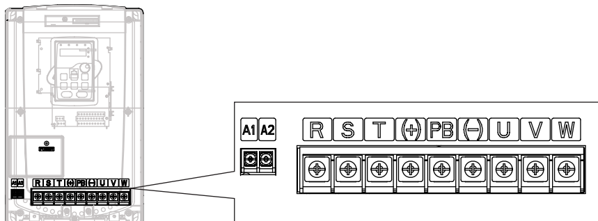
Рис. 4-12 22~30 кВ клеммы силовых цепей
