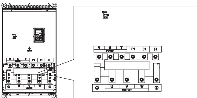
Рис.4-15 132~200 кВт клеммы силовых цепей
