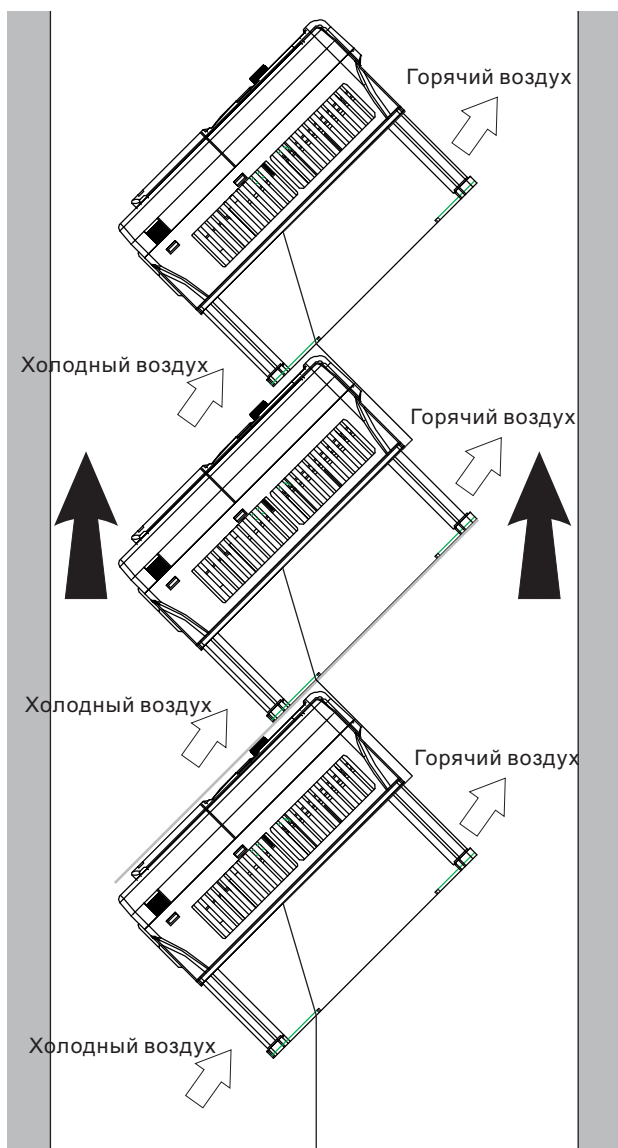
Рис. 4-6 Наклонная установка
