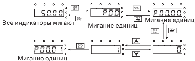
Рис. 5-2 Диаграмма изменения параметров
