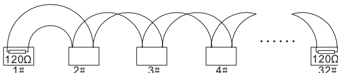
Рис. 10.2 Подключение «Шина»
