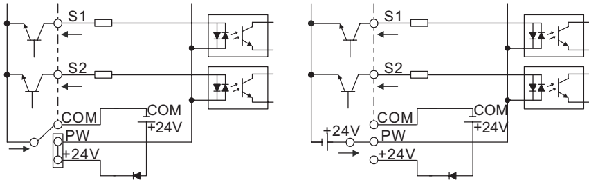
Рис. 4-22 Режим NPN
