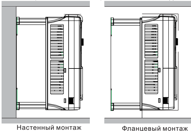
Рис. 4-2 Способ установки
