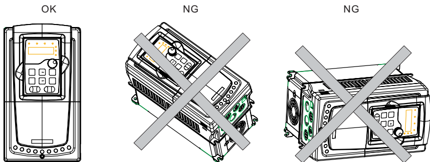
Рис. 4-1 Установка ПЧ
