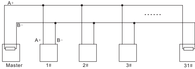
Рис. 10.3 Подключение «Шина»
