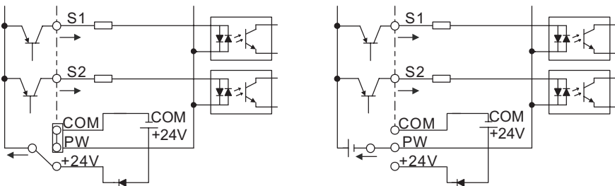
Рис. 4-23 Режим PNP
