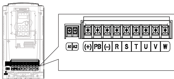
Рис. 4-11 15~18 кВ клеммы силовых цепей
