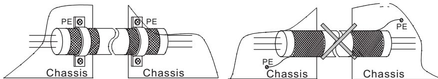
Рис 4-18 Техника заземления 360 градусов
