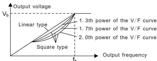
Рис. 7.4. Кривые U/F
