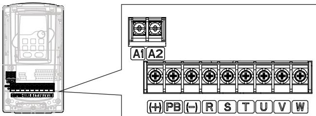
Рис. 4-9 4~9 кВ клеммы силовых цепей
